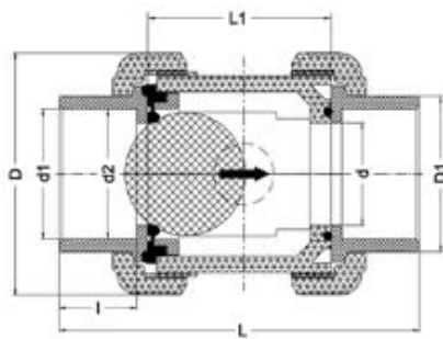
Обратный клапан шаровой с муфтовыми окончаниями PP-H IPS (FKM) d50
