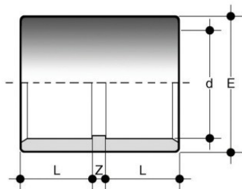
Муфта соединительная ПВХ FIP d125
