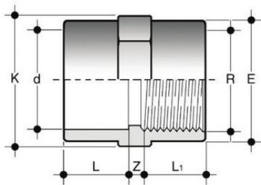
Муфта переходная с ВР ПВХ FIP 50x1 1/2
