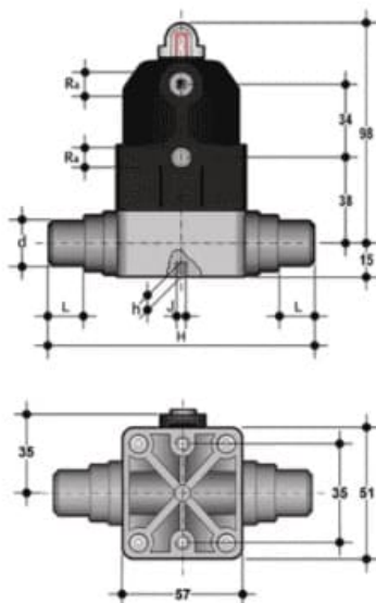
Компактный мембранный клапан CM с пневмоприводом НЗ с муфтовыми окончаниями (уплотнение EPDM/мембрана EPDM) PP-H d16 (DN12)
