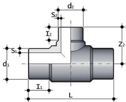
Тройник редукционный для стыковой сварки PP-H FIP 225x110 SDR17.6 PN10
