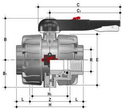
Шаровой кран промышленного применения VKD ХПВХ с резьбовыми окончаниями, DN65-100 R3" (DN80)
