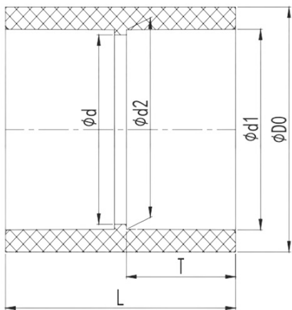
Муфта соединительная ПВХ IPS d25
