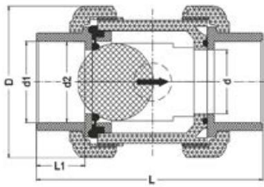
Обратный клапан шаровой с муфтовыми окончаниями PP-H IPS d32
