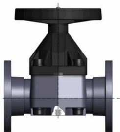
Мембранный клапан VMOV PBX с фланцевыми окончаниями, FKM, FIP d110 (DN100)
