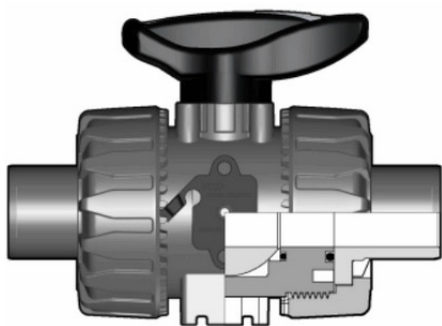
Шаровой кран ПВХ промышленного применения VKD со втулочными окончаниями, EPDM, FIP d40 (DN32)
