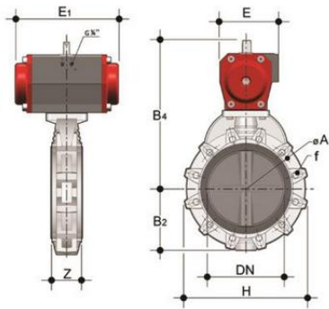
Дисковый затвор FK с пневмоприводом ДвД (уплотнение EPDM) PP-H d250 (DN250)
