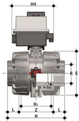
Шаровой кран VKD ПБХ с эл.приводом 24V AC/DC, резьбовые окончания, EPDM, FIP R3" (DN80)
