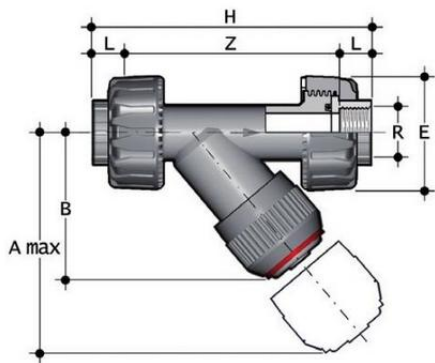
Грязевой фильтр RVUFM с резьбовыми окончаниями (уплотнение FKM) PP-H R1¼" (DN32)
