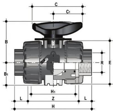
Шаровой кран для регулирования потока VKRFM с резьбовыми окончаниями (уплотнение FKM) PP-H 1¼"
