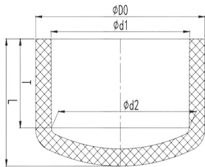
Заглушка клеевая ПВХ IPS d63
