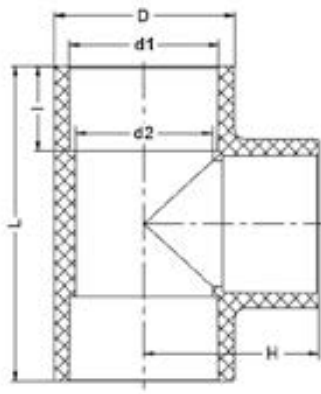
Тройник ПВДФ для раструбной сварки 90° d32 PN 16
