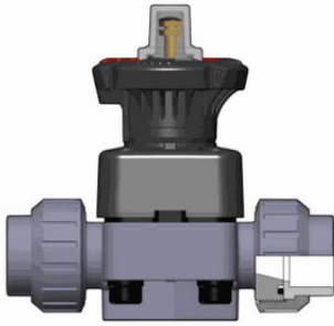
Мембранный клапан DKLUIV ПВХ с разборными муфтовыми окончаниями, EPDM, FIP d25 (DN20)
