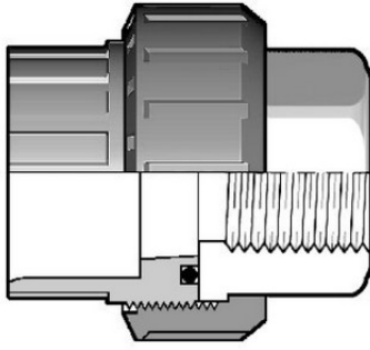
Муфта разборная переходная ХПВХ/ нержавеющая сталь ВР 63x2" PN16
