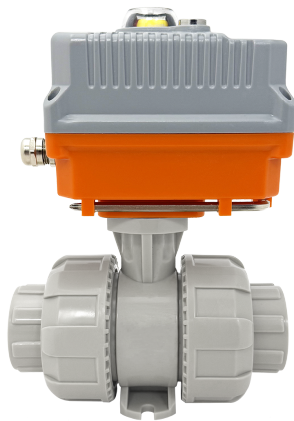
Шаровой кран IVKD ПП-гомополимер с эл.приводом 220V AC, муфтовые окончания, EPDM, IPS d110 (DN100)
