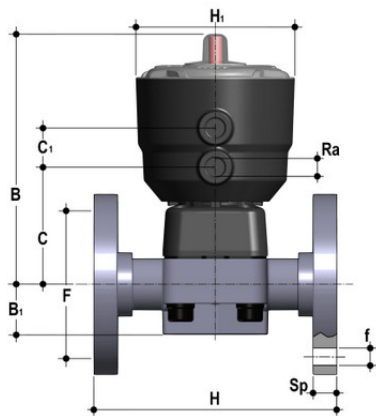
Мембранный клапан ДК ПВДФ с пневмоприводом НЗ, PN10 с фланцевыми окончаниями d20
