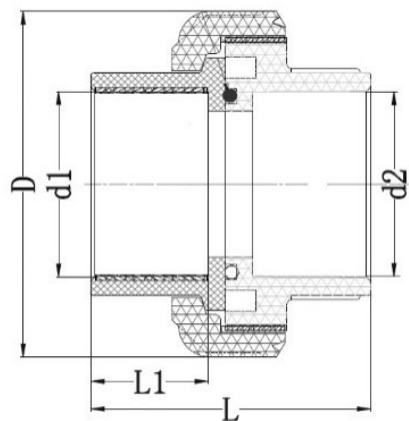
Муфта разборная с ВР, РР-Н IPS d20 PN10
