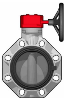
Дисковый затвор FK ПВХФ с редуктором d315 (DN300)
