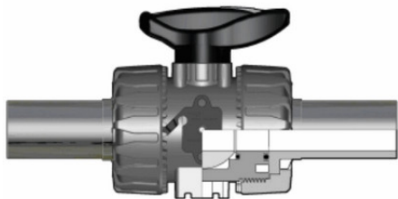
Шаровой кран промышленного применения VKD с патрубками (CVDM) (уплотнение FKM) PP-H d50
