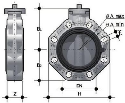
Дисковый затвор ПВХ ФКОAVFM со свободным штоком, ФKM, FIP d14" (DN350)
