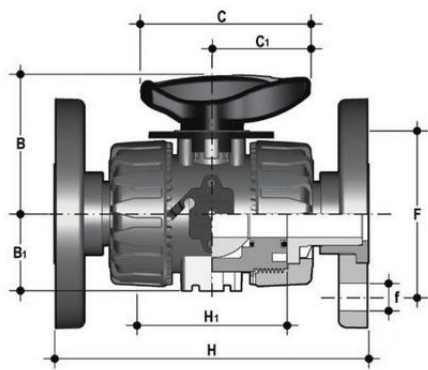
Шаровой кран для регулирования потока VKR ПВДФ с фланцевыми окончаниями d40 (DN32)
