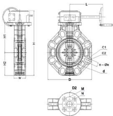
Затвор дисковый ПВХ с редуктором промышленный IPS (Model A) 10"
