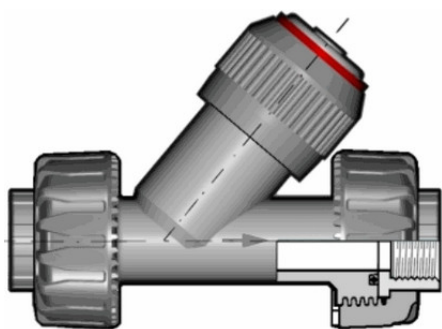
Угловой обратный клапан VRUFV ПВХ с резьбовыми окончаниями, EPDM, FIP R1½" (DN40)
