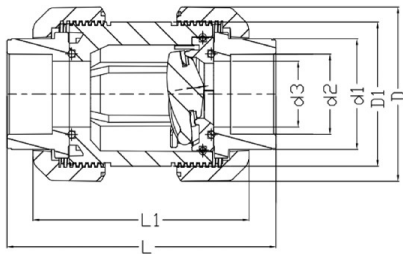
Шаровой обратный клапан ISXE ПВДФ, втулочные окончания d63 (DN50)
