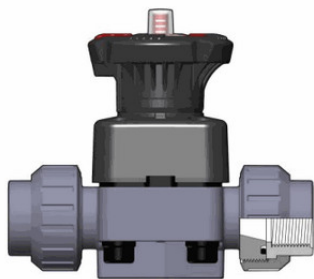
Мембранный клапан DKUFV PBX с резьбовыми окончаниями, FKM, FIP R1" (DN25)
