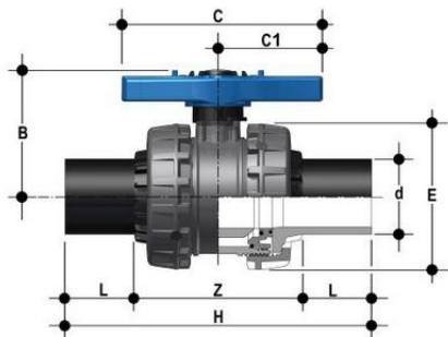
Шаровой кран ПВХ общего применения VEE; муфтовые окончания, EPDM, FIP d75 (DN65)
