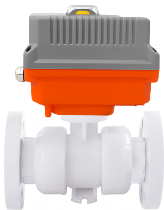
Шаровой кран IVKD ПВДФ с эл.приводом 220V AC, фланцевые окончания, EPDM, IPS d63 (DN50)
