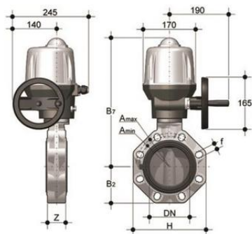
Дисковый затвор FK ПВДФ с эл.приводом 24V AC/DC 12"
