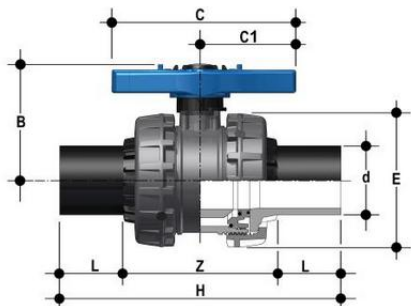
Шаровой кран ПВХ общего применения VEE; муфтовые окончания, EPDM, FIP d110 (DN100)
