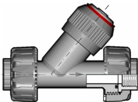
Угловой обратный клапан VRUFV PBX с резьбовыми окончаниями, EPDM, FIP R3/8" (DN10)
