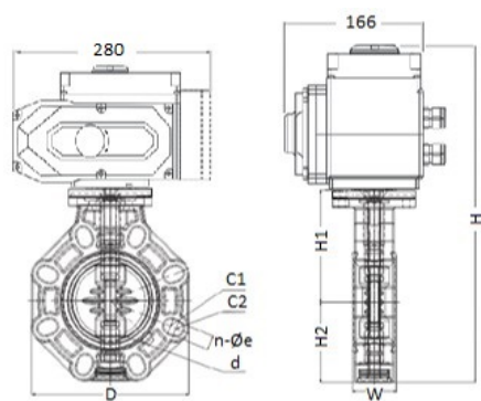
Дисковый затвор IFK PP-H с электрическим приводом 24V DC, FKM, IPS d225 (DN200)
