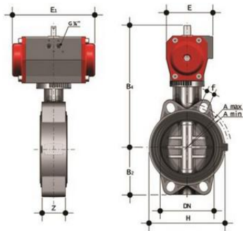
Дисковый затвор общего применения FE ПВХ с пневмоприводом ДвД, FKM, FIP d160 (DN150)
