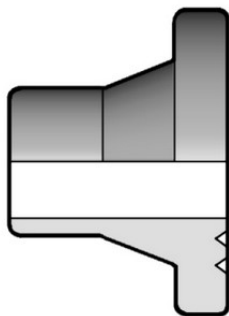
Бурт под фланец для стыковой сварки PP-H FIP (PN10) d315 SDR11 PN10
