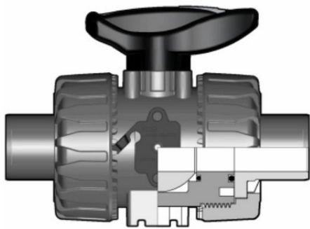
Шаровой кран VKD ПВДФ с втулочными окончаниями d25 (DN20)
