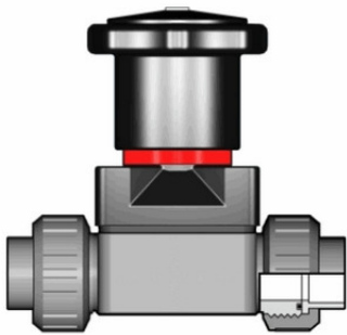
Компактный мембранный клапан CM с разборными муфтовыми окончаниями (уплотнение FKM / мембрана PTFE) PP-H d20 (DN15)
