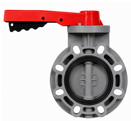
Затвор дисковый в корпусе FRPP (диск — ПП-гомополимер) с рукояткой промышленного применения FKM IPS d110 (DN100)
