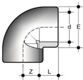
Отвод 90° ХПВХ d32 PN16
