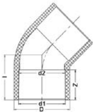
Отвод 45° ХПВХ IPS (Model B) d355 PN10
