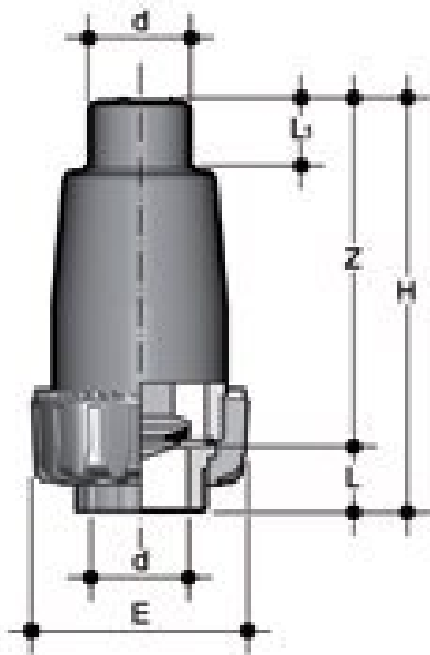
Донный клапан VZIV ПВХ с муфтовыми окончаниями, EPDM, FIP d50 (DN40)
