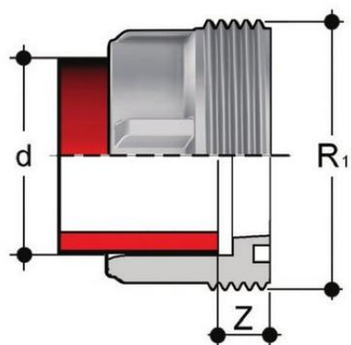
Муфтовая вставка для раструбной сварки PP-H FIP PN10
