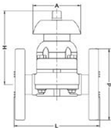
Мембранный клапан IDK PBX с фланцевыми окончаниями, PTFE, IPS d90 (DN80)
