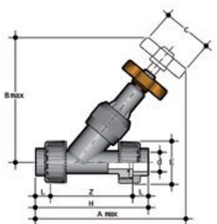
Угловой вентиль VVUIV ПВХ с разборными муфтовыми окончаниями, EPDM, FIP d63 (DN50)
