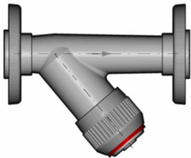
Грязевый фильтр RVOT ПВХ с фланцевыми окончаниями, EPDM, FIP d63 (DN50)
