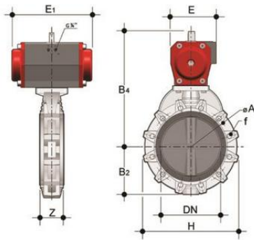
Дисковый затвор FK с пневмоприводом ДвД (уплотнение EPDM) PP-H d315 (DN300)
