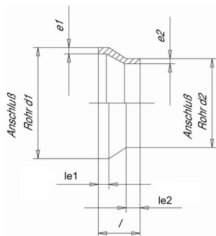
Муфта редукционная ПВДФ (Simona) 140x110 SDR33 PN10
