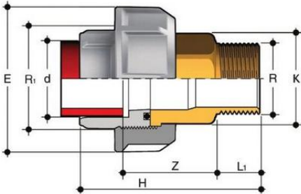
Муфта разборная переходная PP-H / латунь, HP (EPDM) FIP 63x2 PN10
